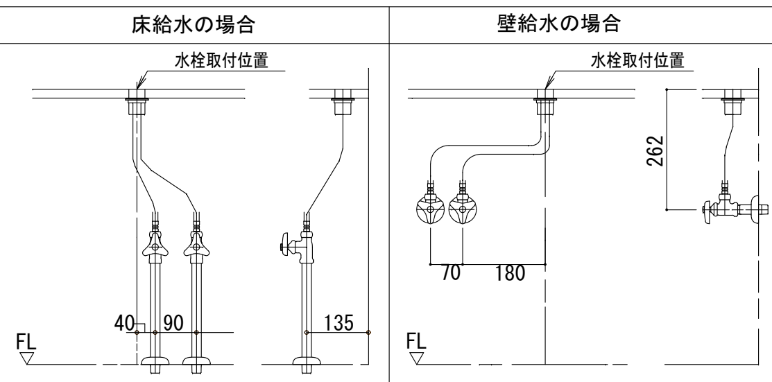
止水栓 (別途手配) 参考位置
