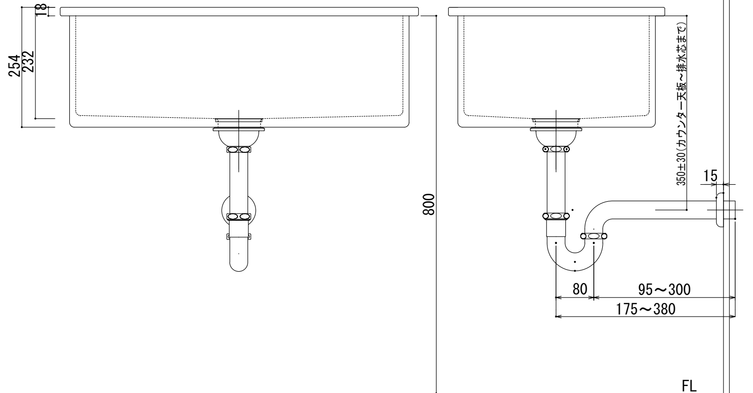
Pトラップ仕様
